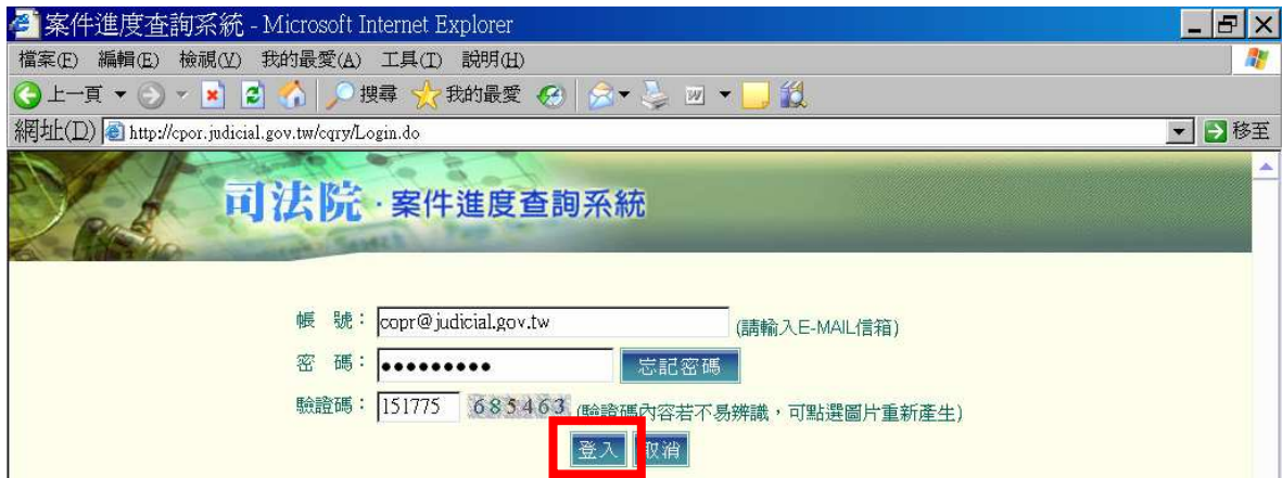
圖 8.1 登入系統
