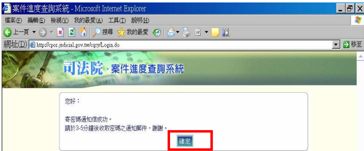
圖 9.2 按「確定」
